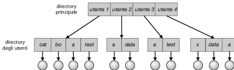
Figura 13.8 Struttura della directory a due livelli.
