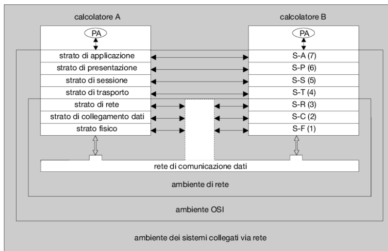
Figura 19.5 Due calcolatori comunicanti attraverso il modello di rete OSI.
