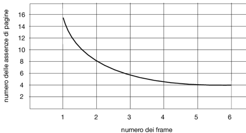
Figura 10.11 Grafico che illustra il numero di page fault rispetto al numero dei frame.
