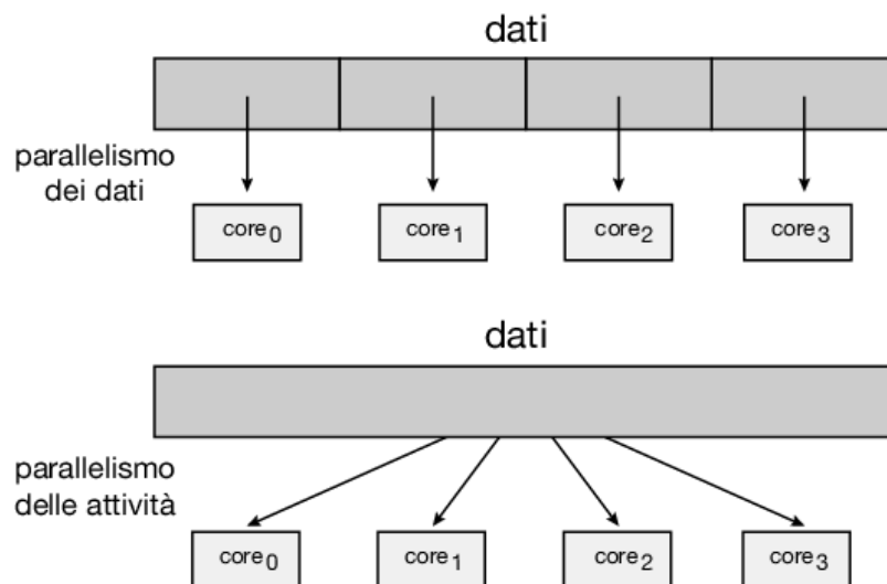
Figura 4.5 Parallelismo dei dati e delle attività.
