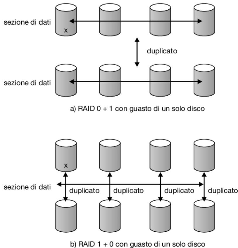
Figura 11.16 raid 0 + 1 e 1 + 0 con guasto di un solo disco.
