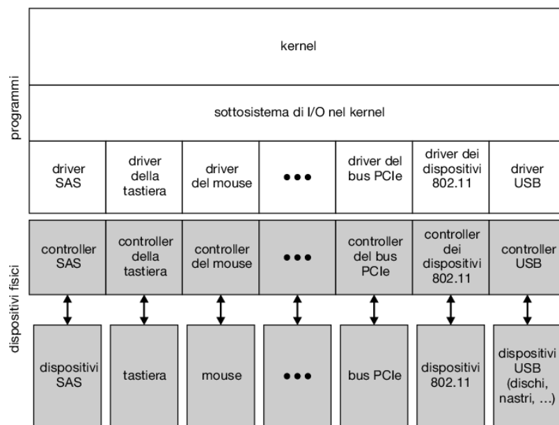
Figura 12.7 Struttura relativa all'i/o nel kernel.
