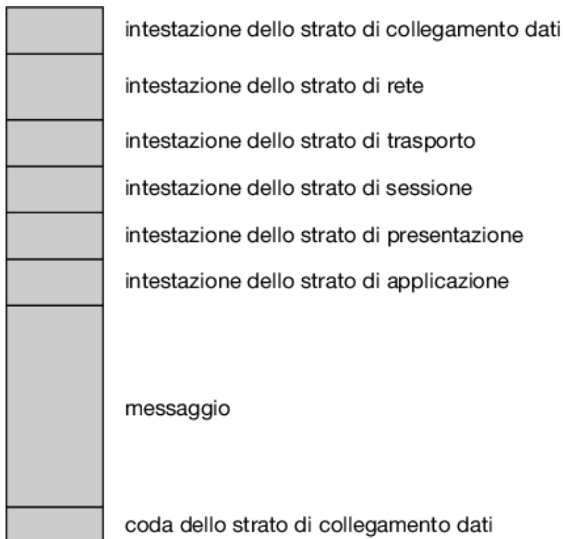
Figura 19.7 Messaggio di rete osi.
