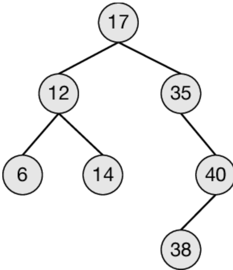
Figura 1.20 Albero binario di ricerca.
