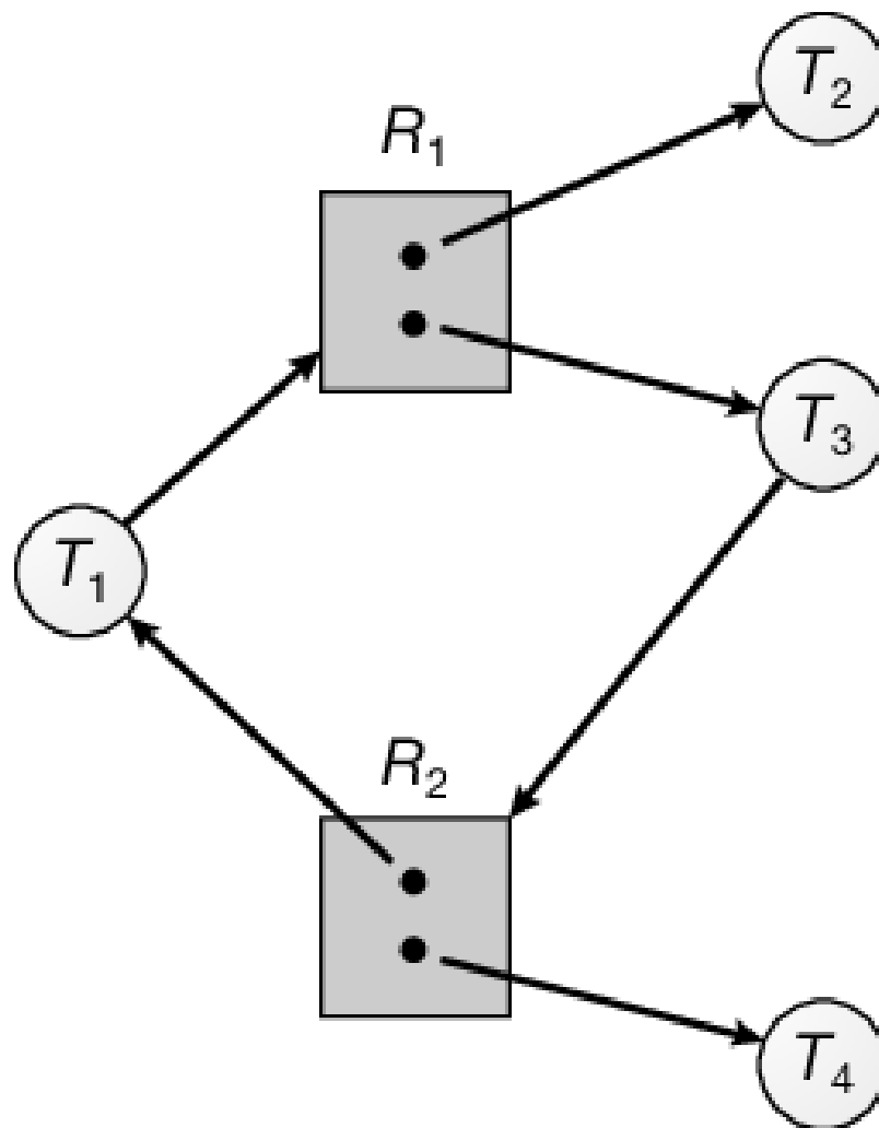
Figura 8.6 Grafo di assegnazione delle risorse con un ciclo, ma senza stallo.
