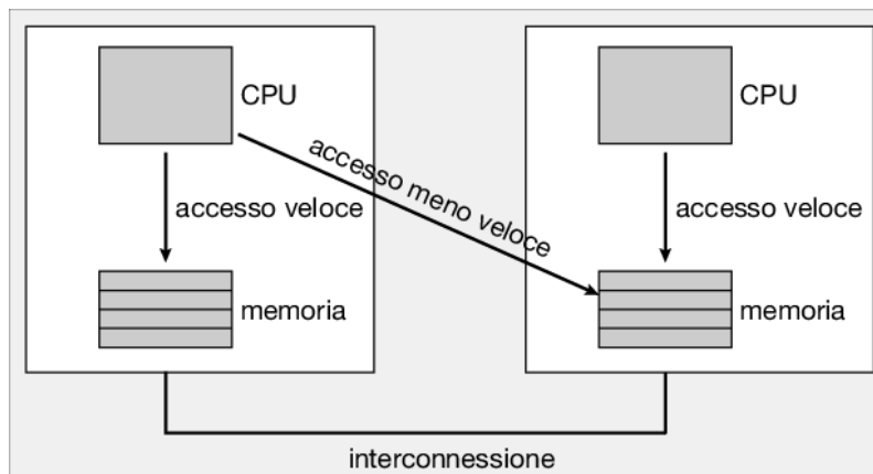
Figura 5.16 numa e lo scheduling della cpu.
