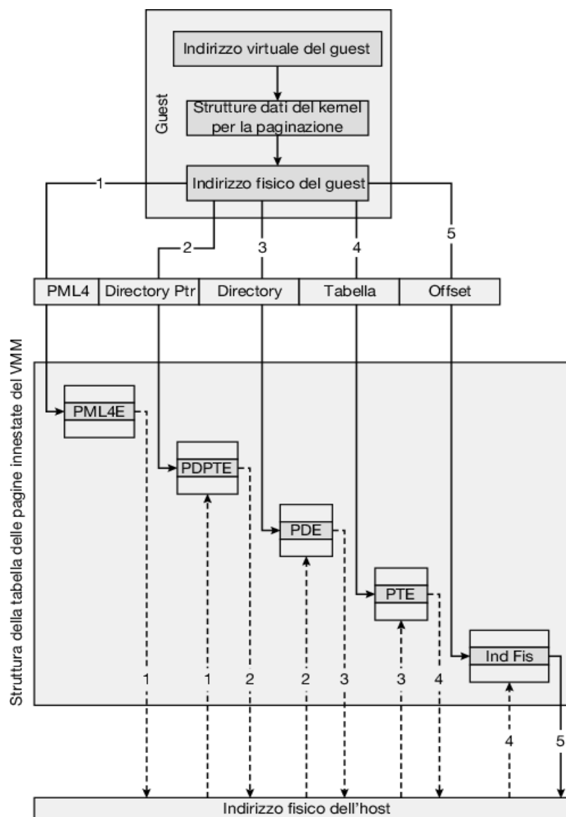
Figura 18.4 Tabelle delle pagine innestate.
