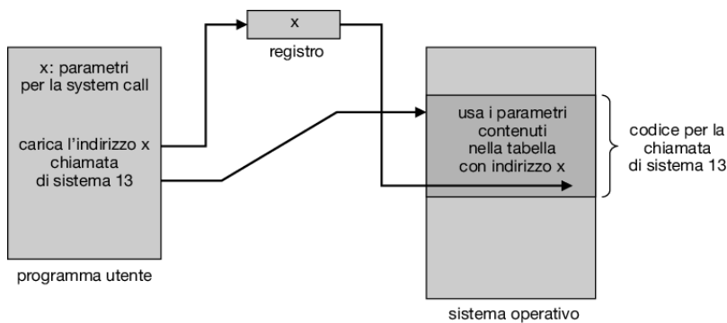
Figura 2.7 Passaggio di parametri in forma di tabella.
