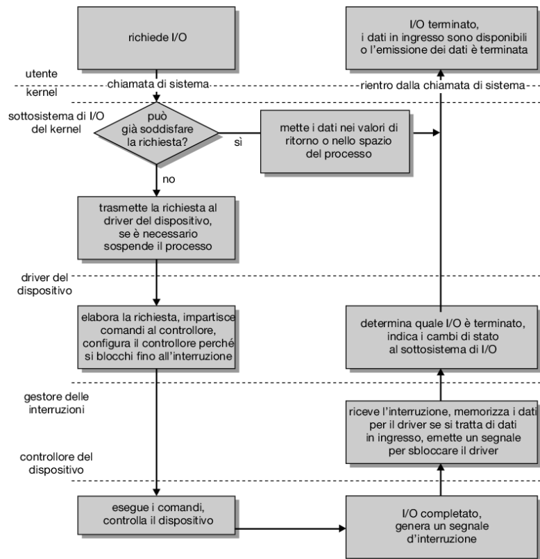
Figura 12.14 Schema d'esecuzione di una richiesta di i/o.
