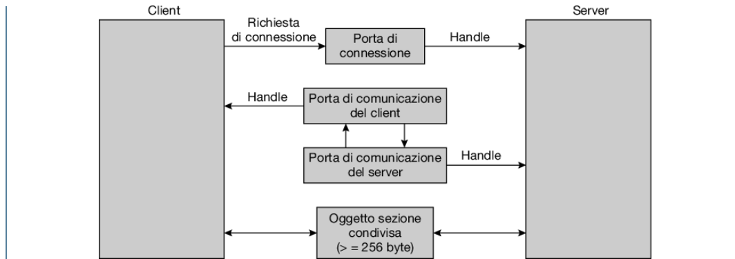
Figura 3.19 Chiamate di procedura locale avanzate in Windows.
