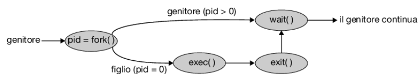
Figura 3.9 Creazione di un processo utilizzando la chiamata di sistema fork() .
