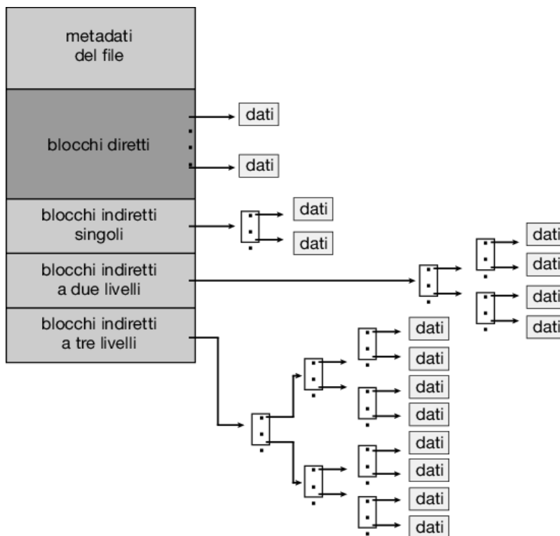
Figura 14.8 Inode di unix.
