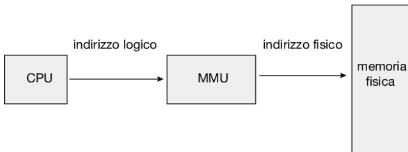
Figura 9.4 Unità di gestione della memoria (MMU).
