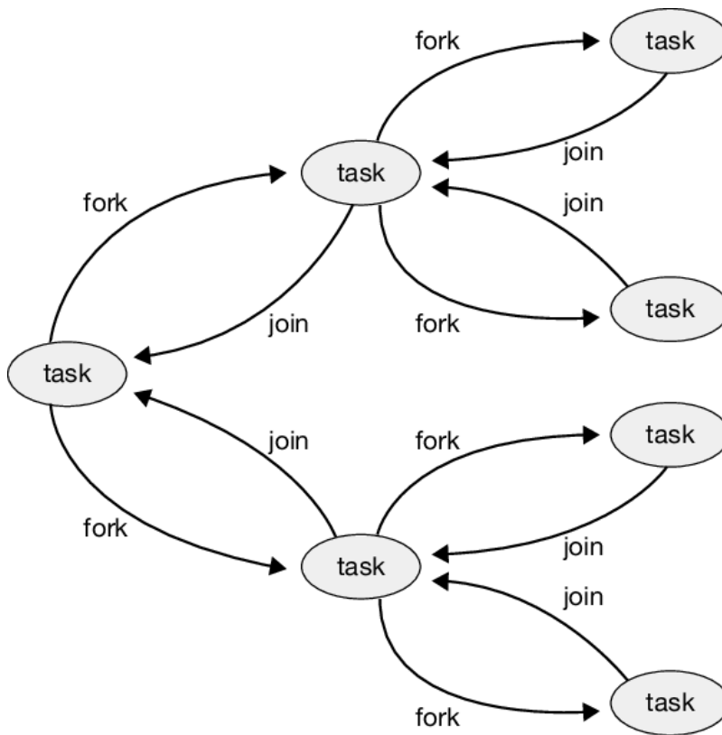
Figura 4.17 Fork-join in Java.
