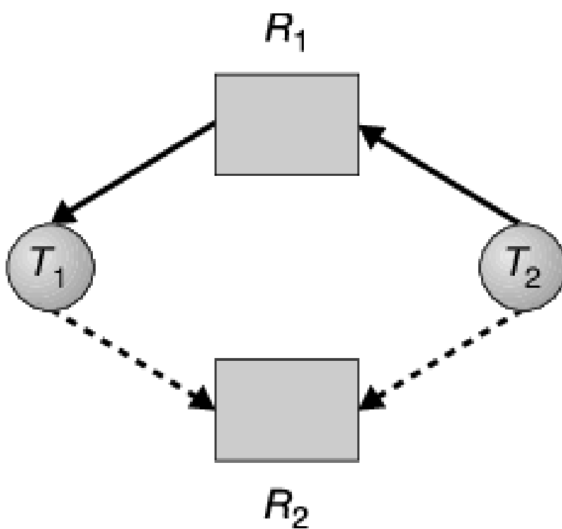
Figura 8.9 Grafo di assegnazione delle risorse per evitare le situazioni di stallo.
