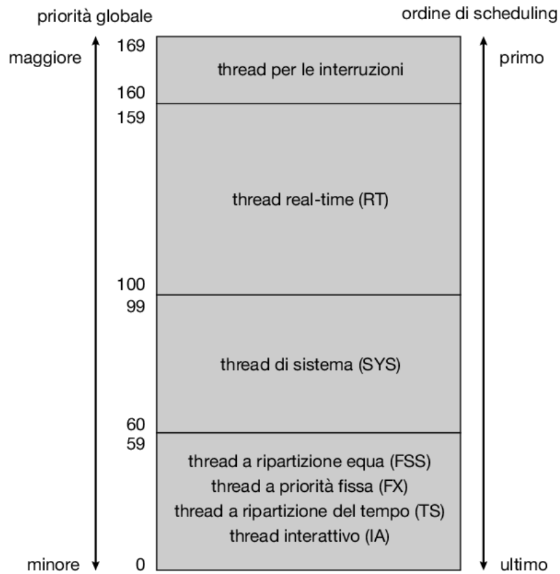
Figura 5.30 Scheduling di Solaris.
