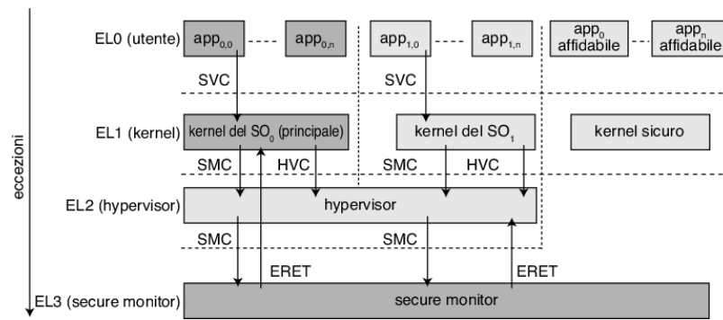
Figura 17.3 Architettura arm.
