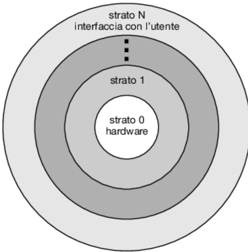
Figura 2.14 Struttura a strati di un sistema operativo.
