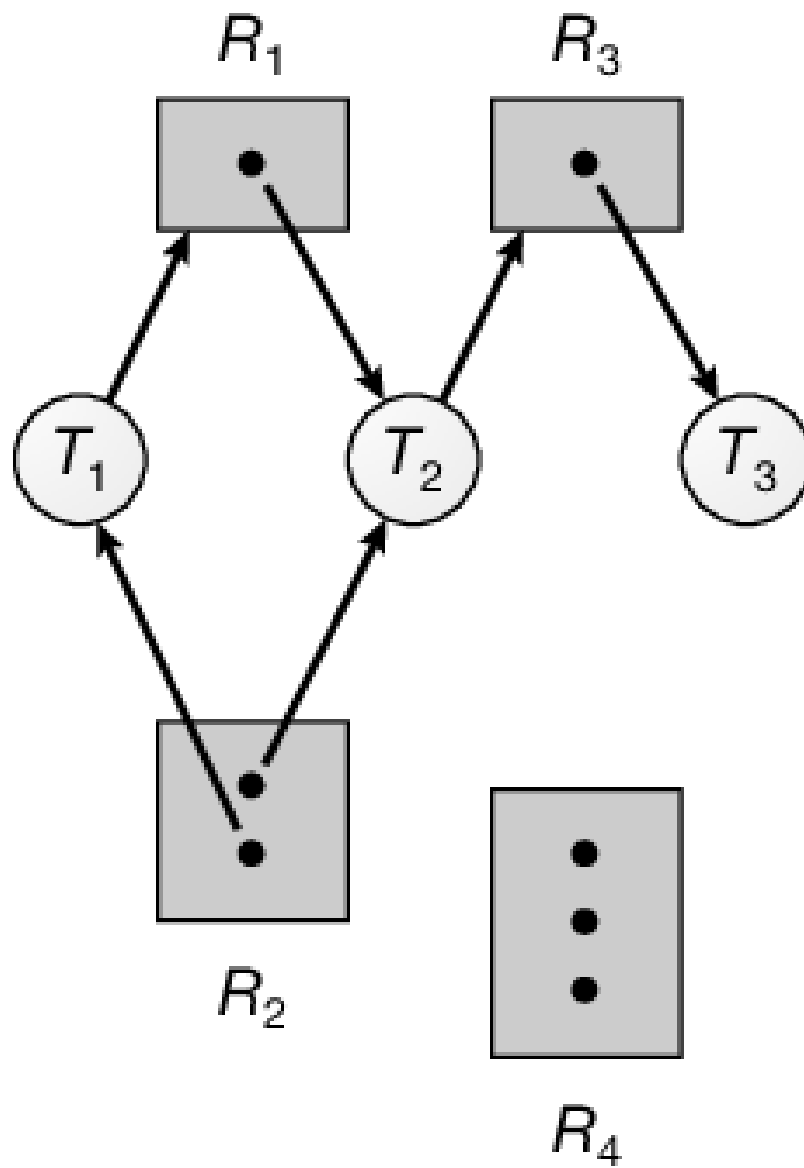
Figura 8.4 Grafo di assegnazione delle risorse.
