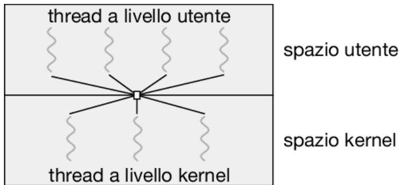
Figura 4.9 Modello da molti a molti.
