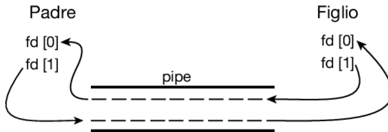
Figura 3.20 Descrittori di file per una pipe convenzionale.
