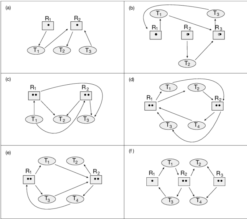
Figura 8.13 Grafici di allocazione delle risorse per l'Esercizio 8.18.
