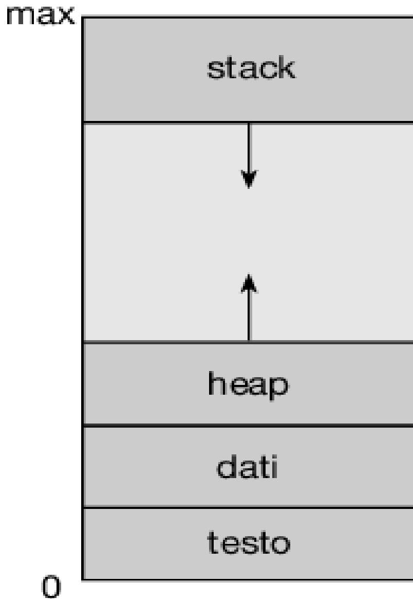
Figura 3.1 Struttura di un processo in memoria.
