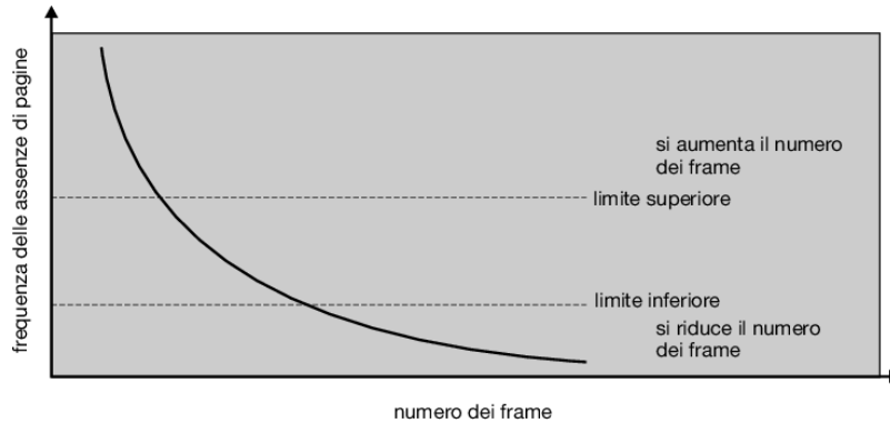
Figura 10.23 Frequenza dei page fault.
