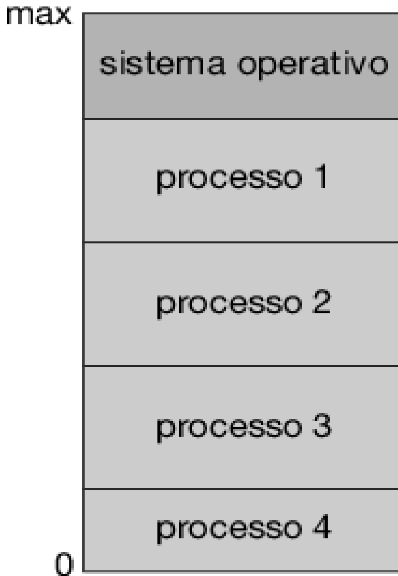
Figura 1.12 Configurazione della memoria per un sistema con multiprogrammazione.
