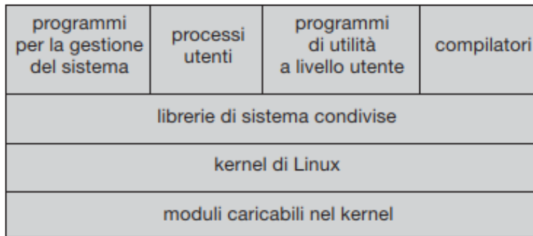
Figura 20.1 Componenti del sistema Linux.
