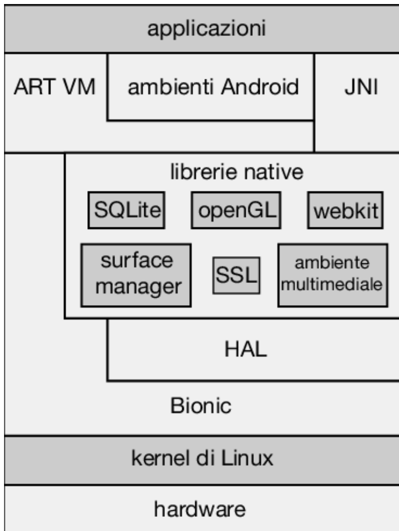
Figura 2.18 Architettura di Google Android.
