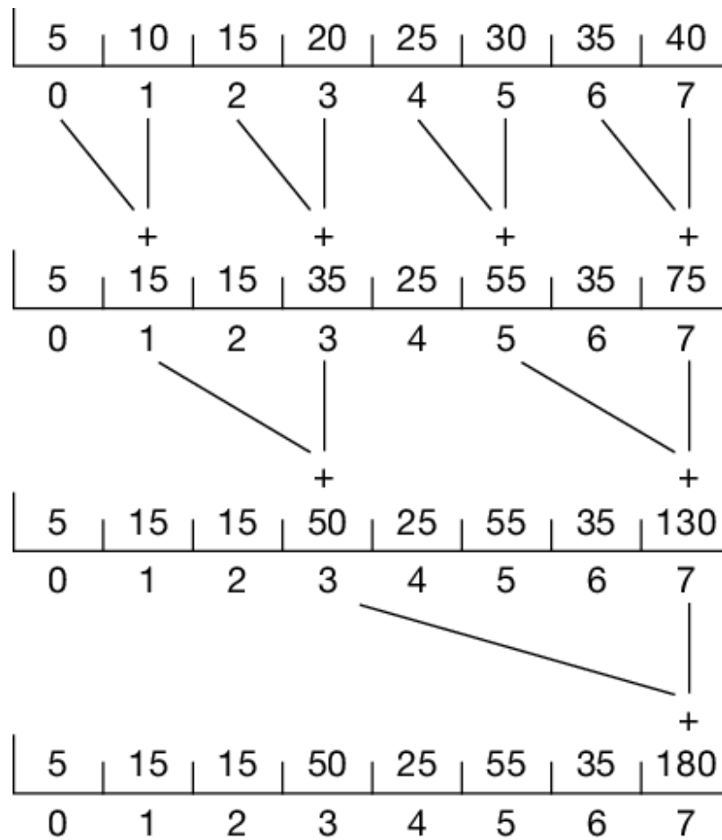
Figura 6.16 Somma di un array come serie di somme parziali per l'Esercizio 6.9.
