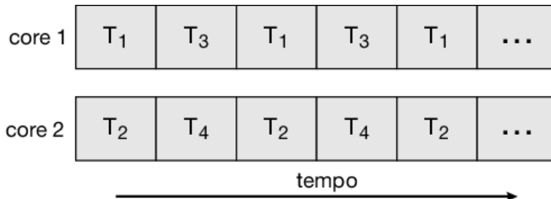
Figura 4.4 Esecuzione parallela su un sistema multicore.
