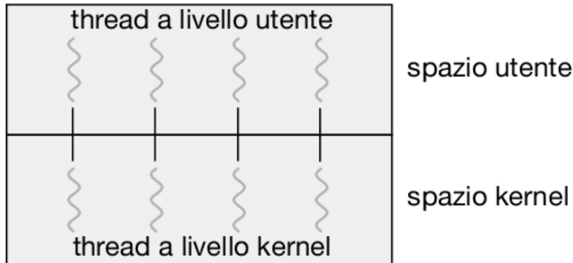
Figura 4.8 Modello da uno a uno.
