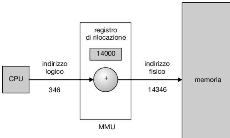
Figura 9.5 Rilocazione dinamica tramite un registro di rilocazione.
