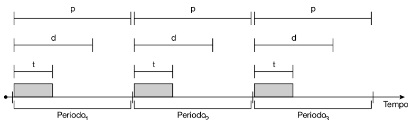
Figura 5.20 Processo periodico.
