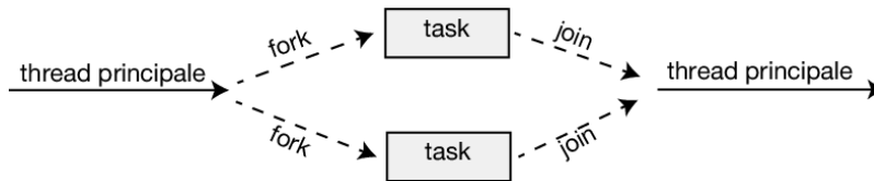
Figura 4.16 Parallelismo fork-join.
