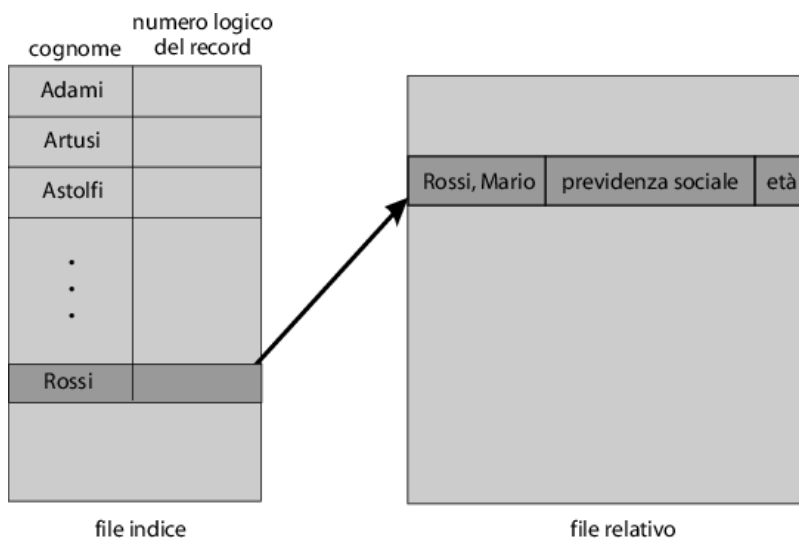
Figura 13.6 Esempio di indice e relativi file.
