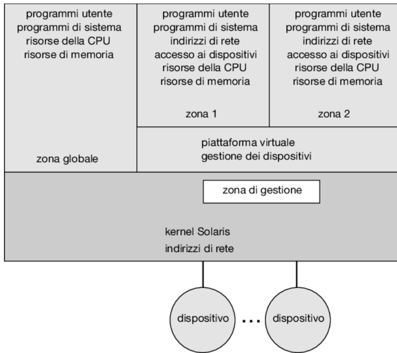
Figura 18.7 Solaris 10 con due zone.
