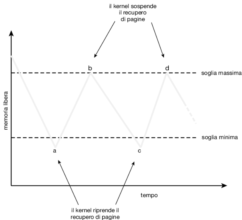
Figura 10.18 Recupero di pagine.
